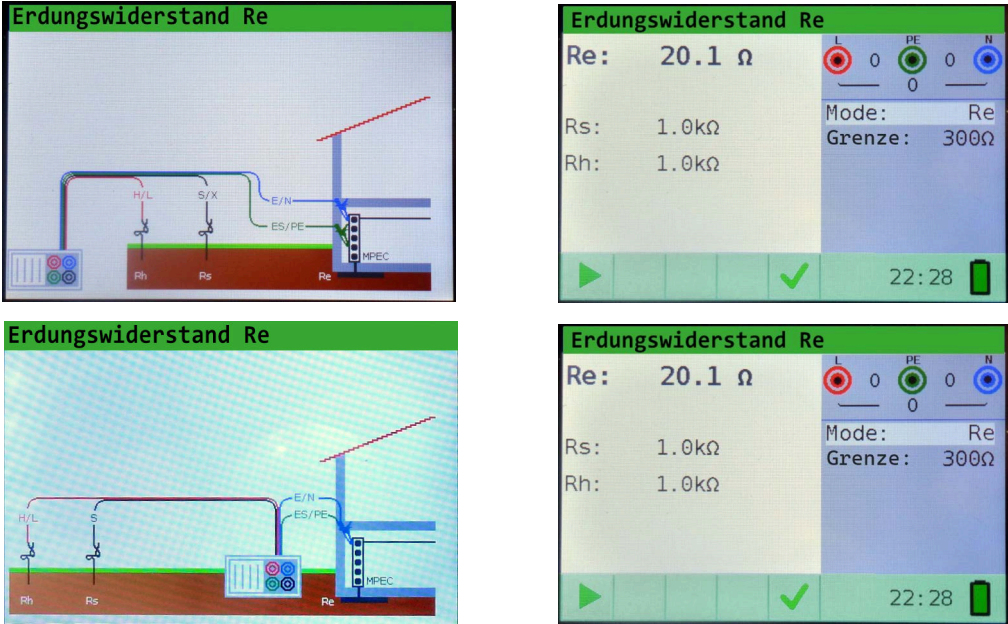
Abb. 21: Erdwiderstandsmessung, Kabelanschluss und Ergebnisse
