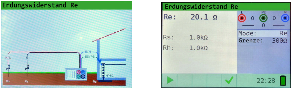
Abb. 21: Erdwiderstandsmessung, Kabelanschluss und Ergebnisse
