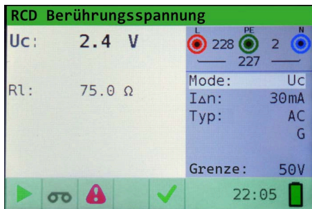
Abb. 10: Messung der Kontaktspannung, Kabelanschluss und Ergebnisse
