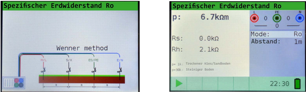
Abb. 22: Messung des spezifischen Erdwiderstands Ro, Kabelanschluss und Ergebnisse
