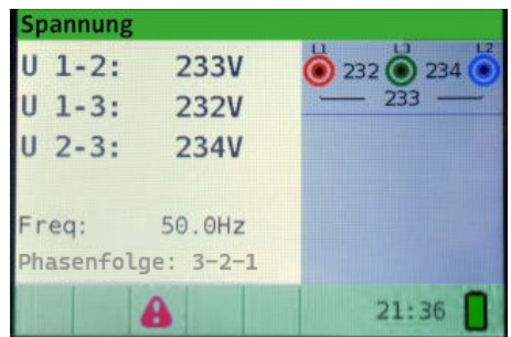
Abb. 20: Spannungs- und Frequenzmessung, Kabelanschluss und Ergebnisse
