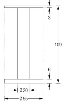
VRH1 Draufsicht:
