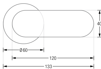
VRH2 Frontansicht:
