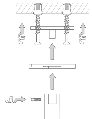
Montage VRH2 mit Rosette:
