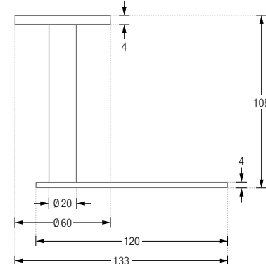
VRH2 Draufsicht:
