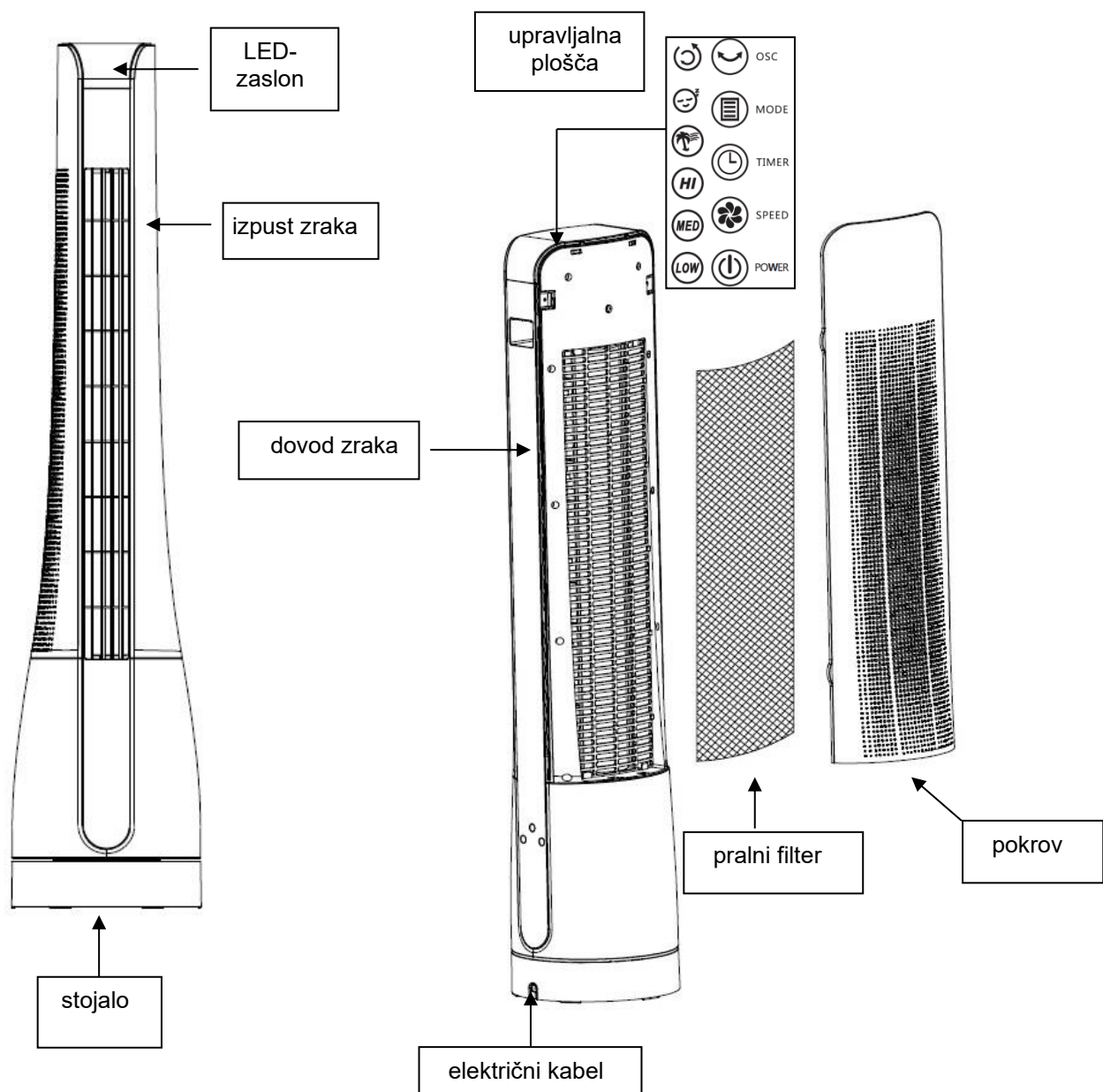
Sprednji pogled
