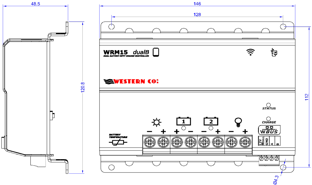
Fig. 5 Dimensions (mm)
