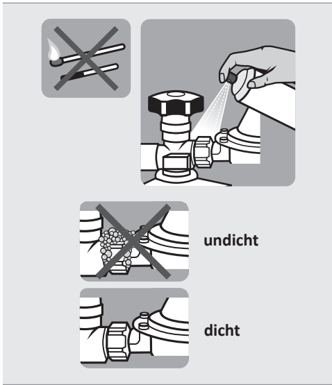
Abb.2: Dichtheitsprüfung
