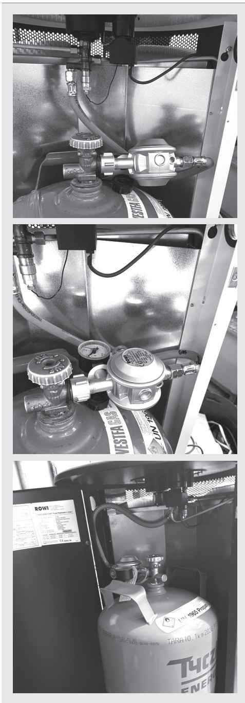
Abb.3b: Verschiedene Installationsmöglichkeiten Gasschlauch (Druckregler am Ende nach vorne drehen, wie in Abb. 3)
