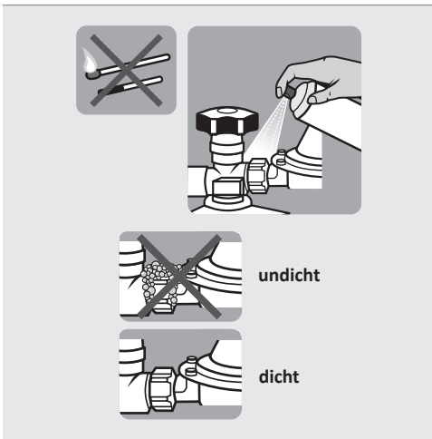
Abb.2: Dichtheitsprüfung
