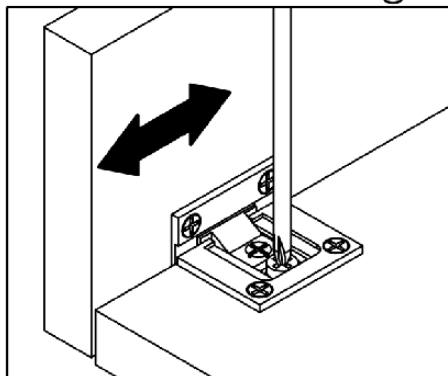
Seitenverstellung
