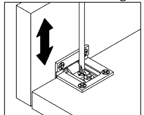
Höhenverstellung
