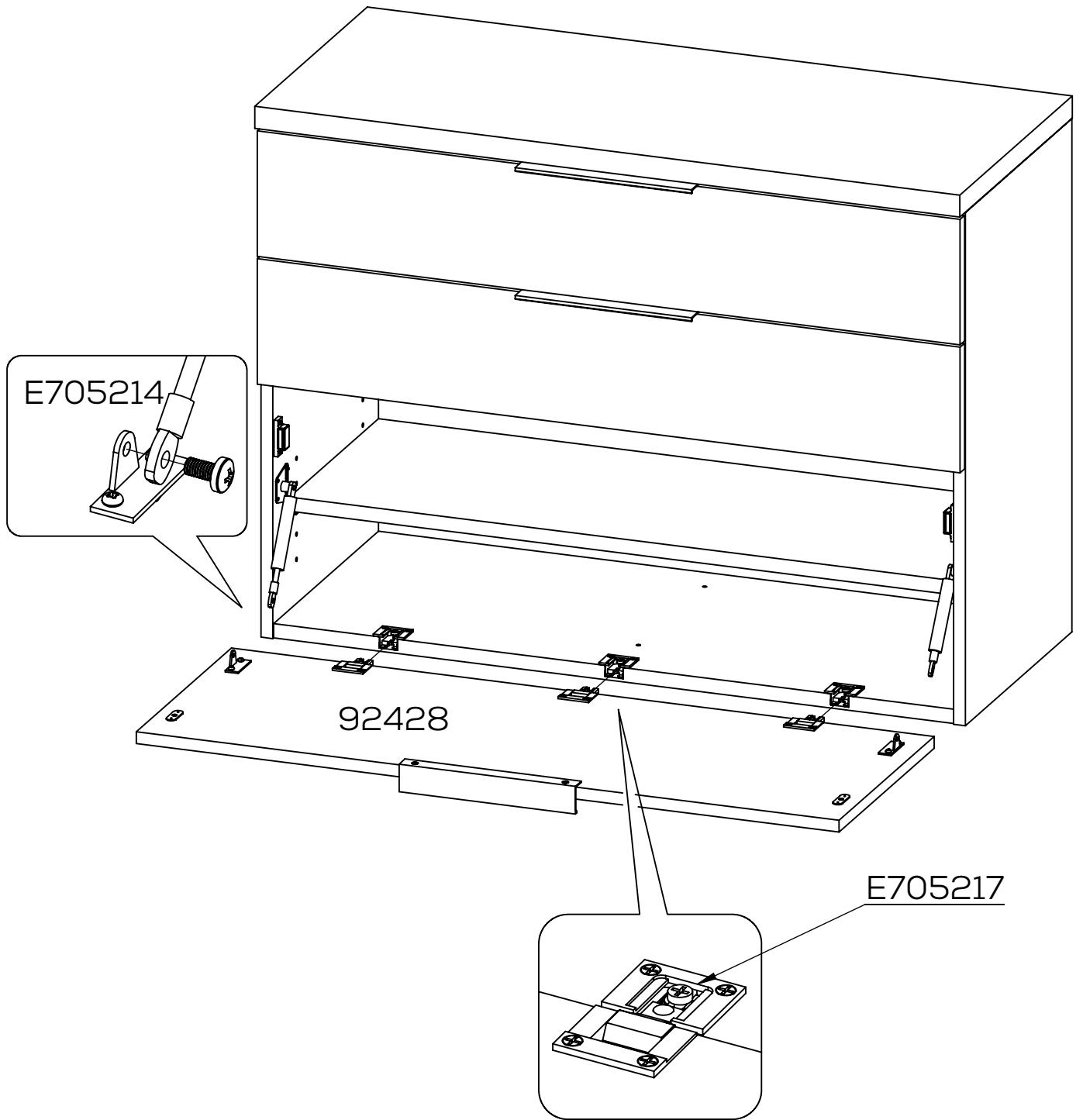
Tiefenverstellung
