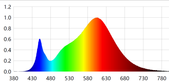
9507 CCT 3000K/6500K(3000K): 1#
