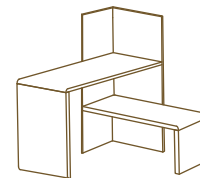
Schreibtisch (74 x 142 x 60 cm) Lowboard (38,8 x 110 x 35 cm) Art.-Nr.: 80 88 01
