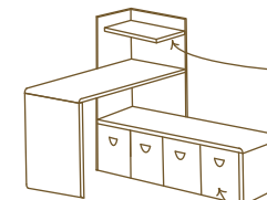
Schreibtisch (74 x 142 x 60 cm) Lowboard (38,8 x 146 x 35 cm) Art.-Nr.: 80 88 02
