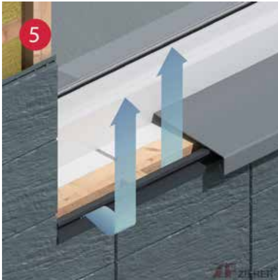
Anschlussprofil der Fassadefläche unter der Fensterbank (Entlüftung).
