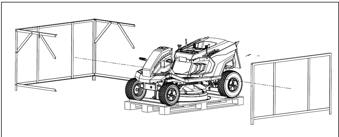
Montage der Heckplatte
