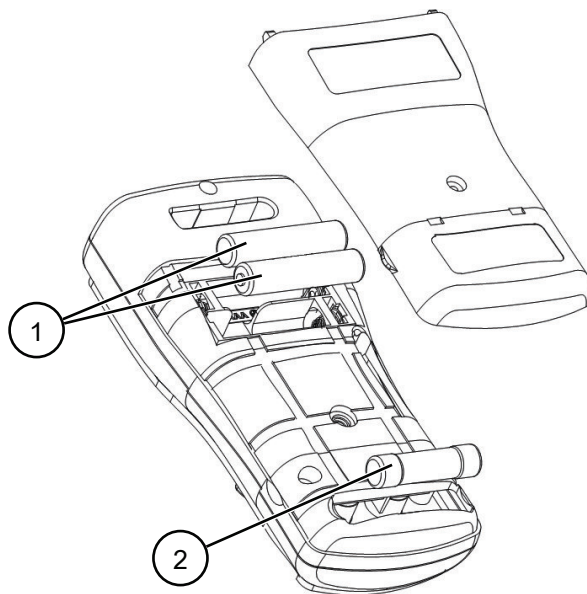
Abb. 16: Batteriewechsel (beispielhaft)
