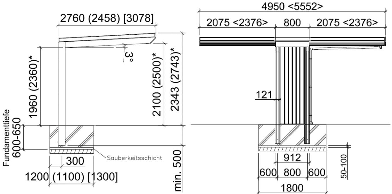
Standard (Sonderbreite XS) [Sonderbreite XL] (Sonderhöhe)*
