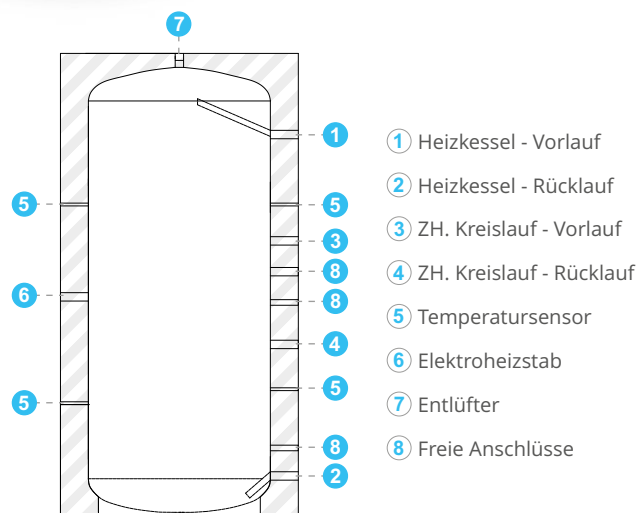
Das Bild zeigt einen 1500 l Pufferspeicher
