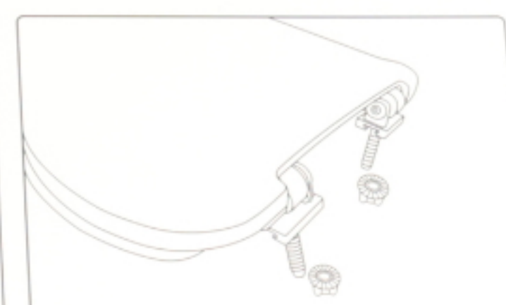
4. Installare Il Coperchio Con Il Dado Fisso Sulla Toilette 4. Instale La Tapa Con La Tuerca Fija Al Inodoro
