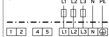
3/N/PE Boilerschaltung - 4 7,5 kW
