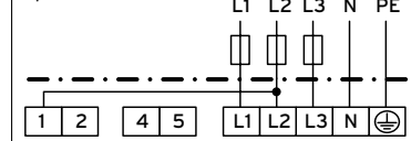
3/N/PE Einkreisumschaltung - 5 7,5 kW
