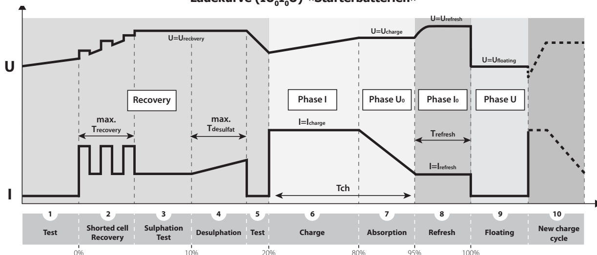
Ladekurve (I U , I 0 , U) «Starterbatterien»
