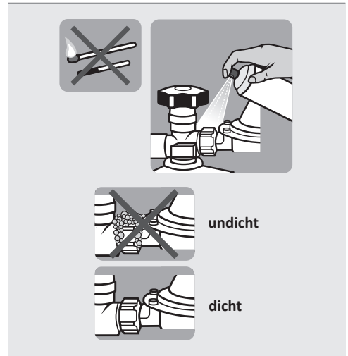
Abb.2: Dichtheitsprüfung
