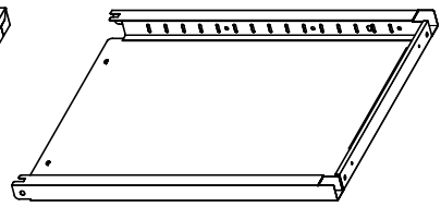
2 Seitenteil 2x
