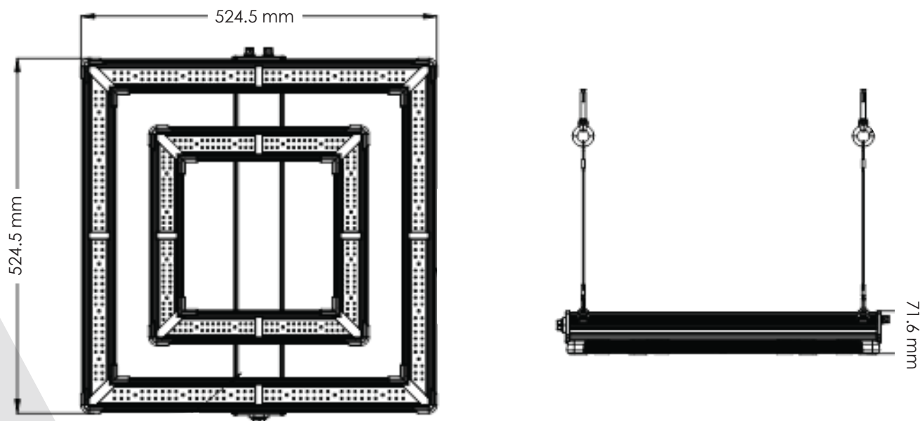
Obr 1. Rozměry svítidla
