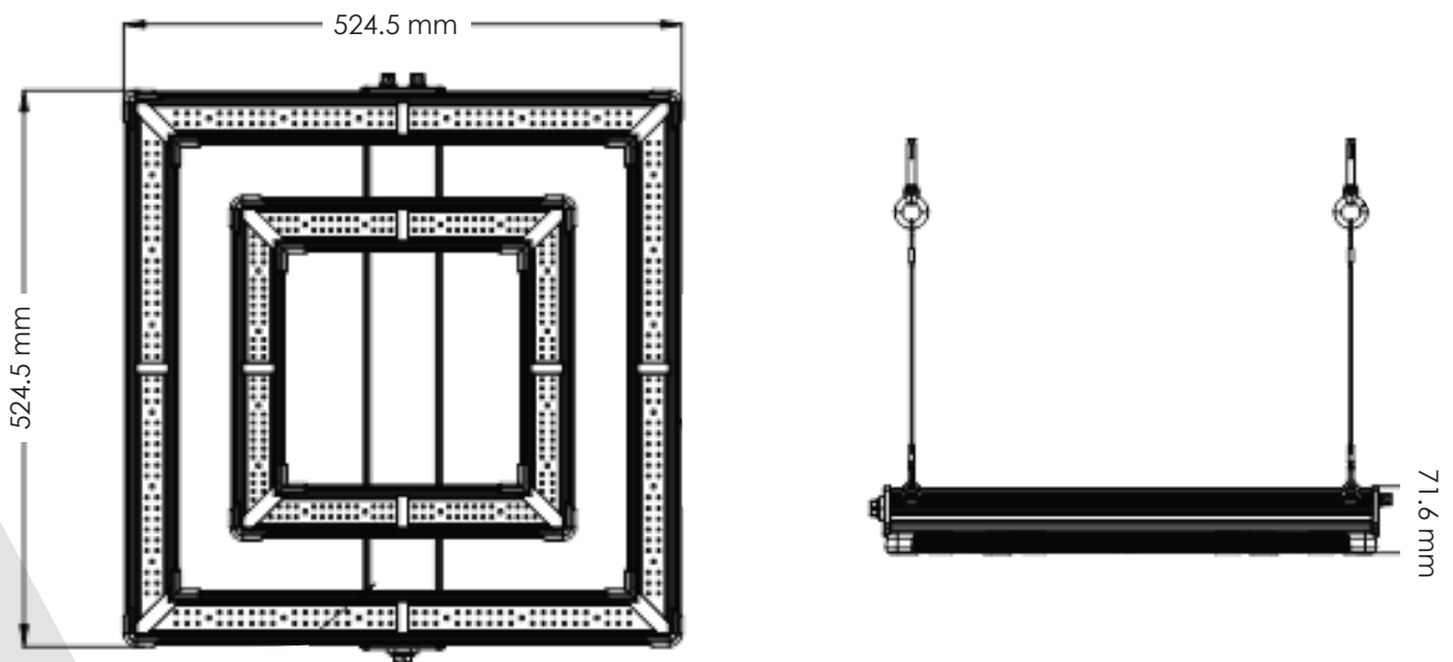
Abb 1. Abmessungen der Halterung
