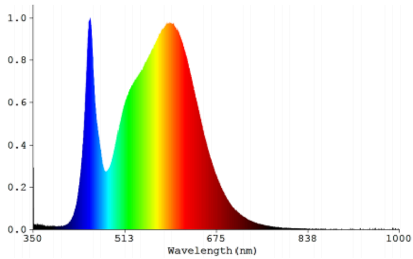
SMD2835-12C5B-0.5M-40
