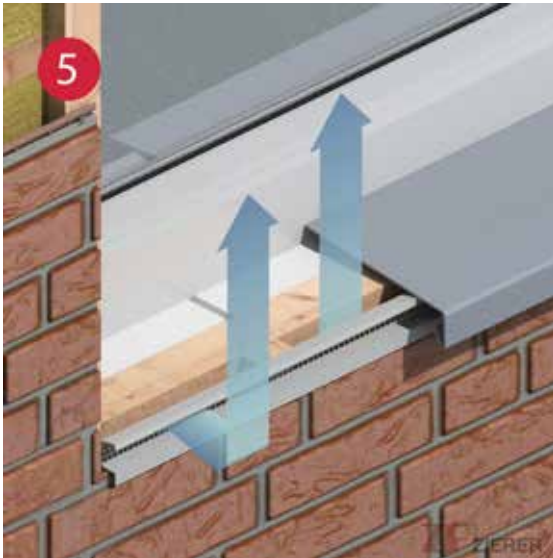
Anschlussprofil der Fassadenfläche unter der Fensterbank (Entlüftung).
