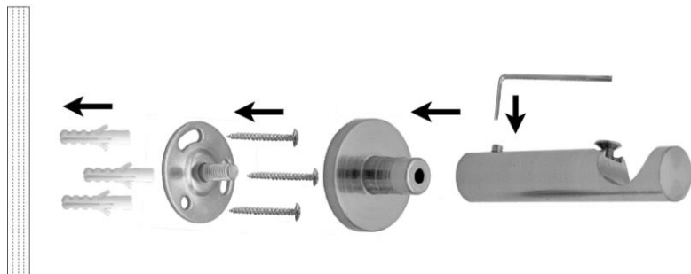
Abbildung 1: Wandträger H10 / H12 / H19
