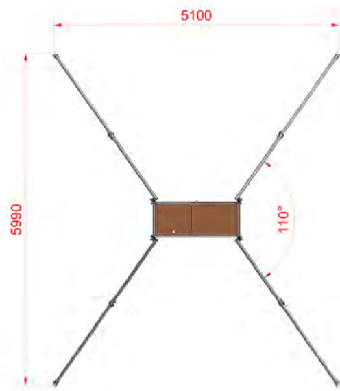
Draufsicht
