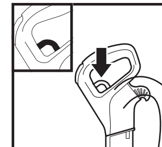
RIMOZIONE DEL MANICO
