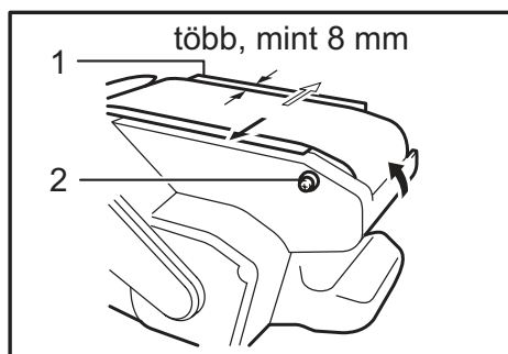
1. Acéllemez 2. Beállítócsavar
