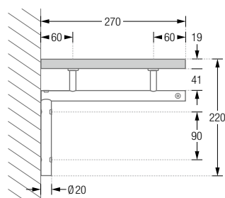
G13-Eiche Seitenansicht:
