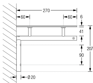
G13-G Seitenansicht:
