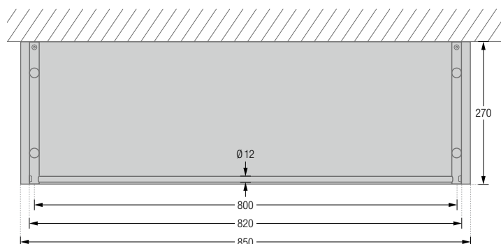
Produktbeispiel G13-800G Draufsicht:
