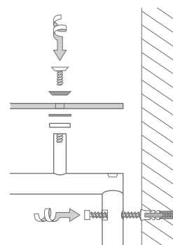
Montage G13-G:
