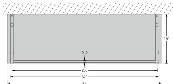
Produktbeispiel G13-800-Eiche Draufsicht:
