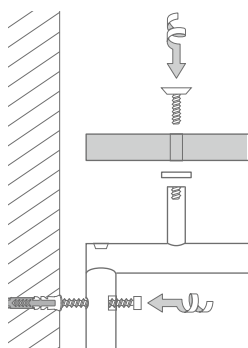
Montage G13-Eiche:
