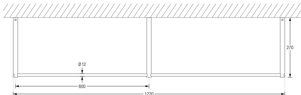
Produktbeispiel G13-1200 Draufsicht:
