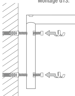
Montage G13:
