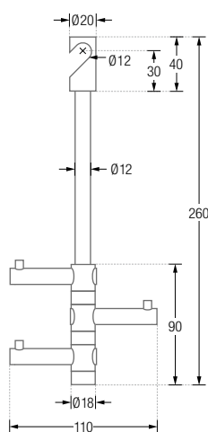
T3H Seitenansicht:
