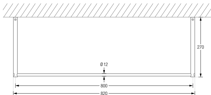
Produktbeispiel G13-800 Draufsicht:
