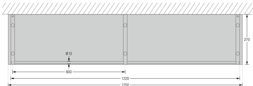
Produktbeispiel G13-1200G Draufsicht:
