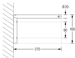
G13 Seitenansicht:
