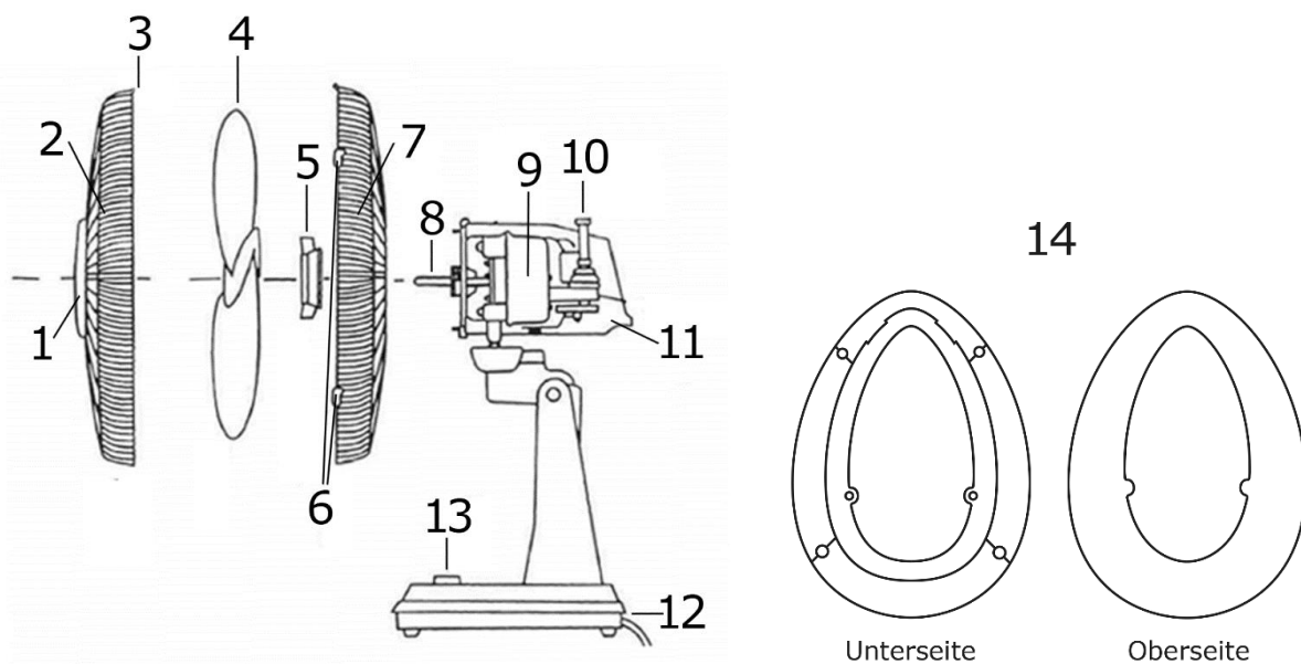
Afbeelding 2 leveringsomvang
