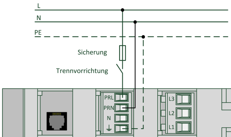
Abbildung 6: Anschluss Versorgungsspannung
