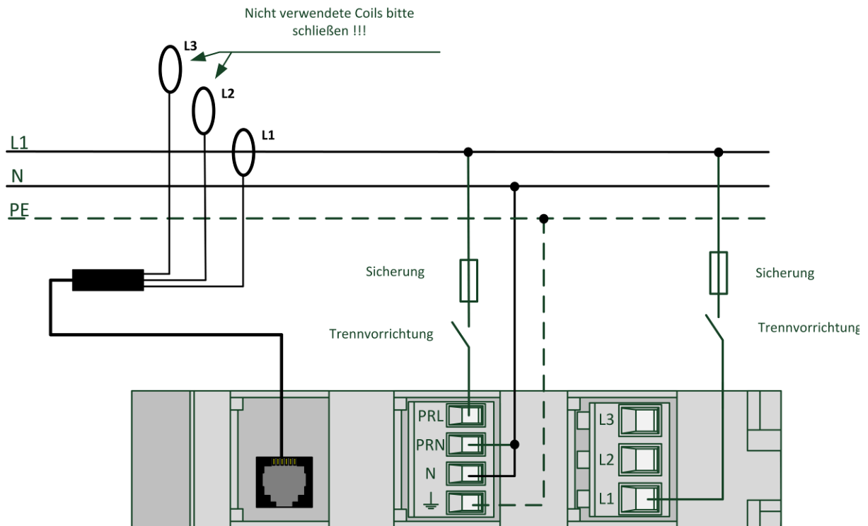
Abbildung 25: 1-Phasen System
