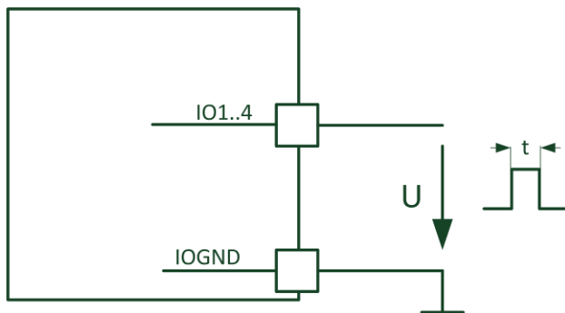
Abbildung 15: Impulseingang
