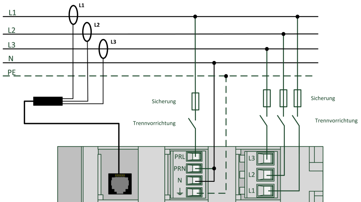
Abbildung 23: 3-Phasen/4-Leiter System beliebiger Belastung
