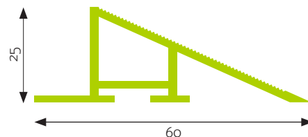
Innenhöhe 25 mm (für Mattenhöhe 22 mm )
