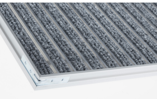
Innenhöhe 10 mm (für Mattenhöhe 8 mm )
