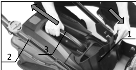
► 1. Hintere Abdeckung 2. Grasfangkorb 3. Griff
