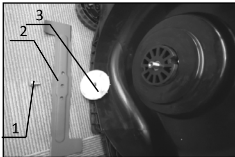
► 1. Sechskantschraube 2. Mähmesser 3. Lüfter
