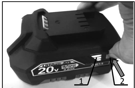
► 1. Anzeigelampen 2. Prüftaste
