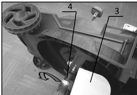
► 1. Mähmesser 2. Sechskantschraube 3. Bauholz 4. Schraubenschlüssel
