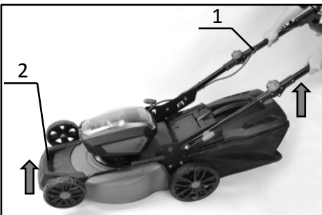
► 1. Unterer Griff 2. Frontgriff
