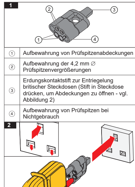
Abbildung 3 zeigt, wie die Prüfspitzen aus der Schutzkappe entnommen bzw. darin verstaut werden.
