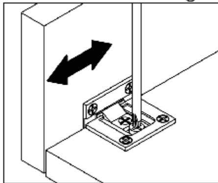
Seitenverstellung
