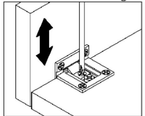
Höhenverstellung
