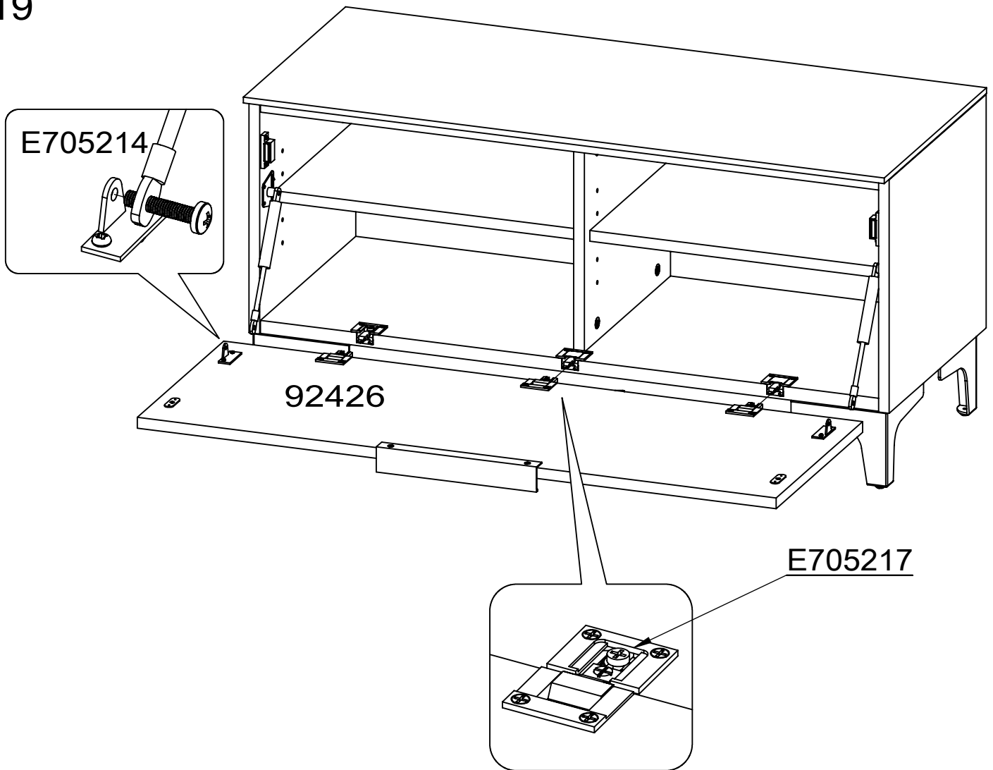
Tiefenverstellung
