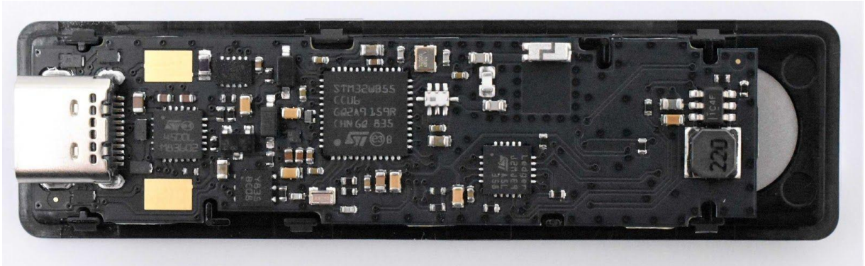
Vorderseite des PCB
