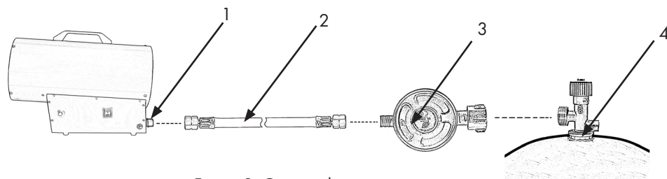
Figuur 3: Gasaansluitsysteem
