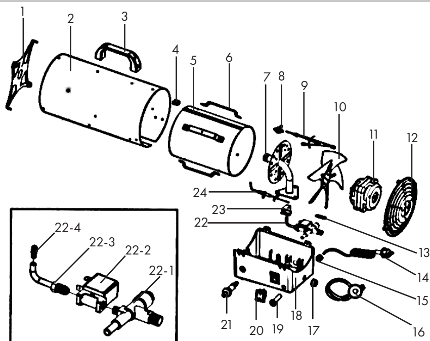
Tabulka 7 Obrázek 13: Obecné součásti zařízení
