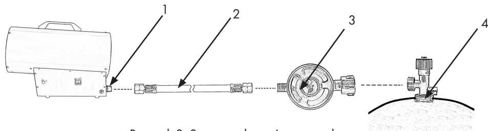
Rysunek 3: System połączeń gazowych
