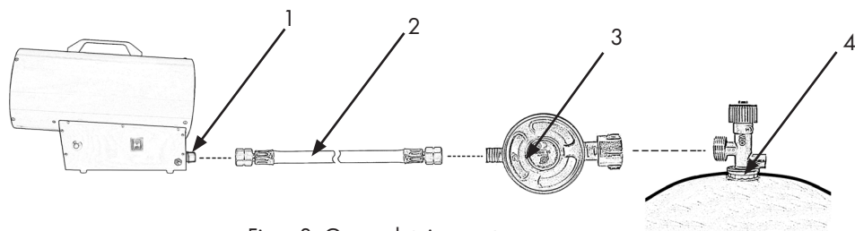
Figur 3: Gasanslutningssystem
