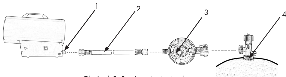
Obrázok 3: Systém pripojenia plynu
