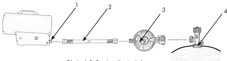
Obrázek 3: Systém připojení plynu
