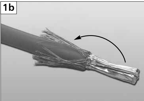
Geflechschirm nach hinten legen ... Fold braided shield backwards ...
