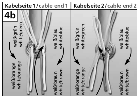
... und nach dem Bild anordnen, um die Adern später leichter in das Ladestück einführen zu können. ... and arrange the pairs as shown on the photos to facilitate insertion to the loader.
