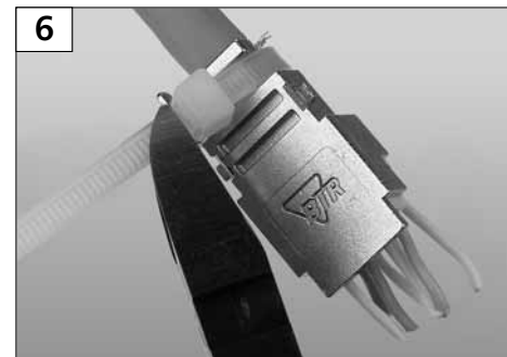
Kabelbinder zur Zugentlastung anbringen und Überlänge entsprechend abschneiden. Fit a cable tie and cut off the excess length.
