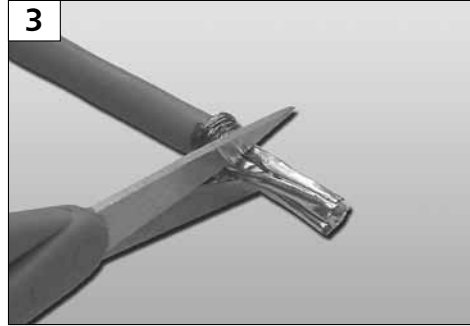
Paar-Schirmfolie einkerben und entfernen. Cut and remove the shield foil of the wire pairs.
