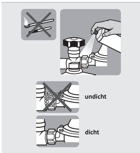
Abb.2: Dichtheitsprüfung
