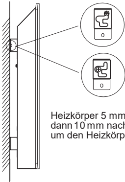
Den Heizkörper von der Wand nehmen
