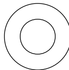
#137. 3/8" × 19 × 1.5T Unterlegscheibe (2 St.)
