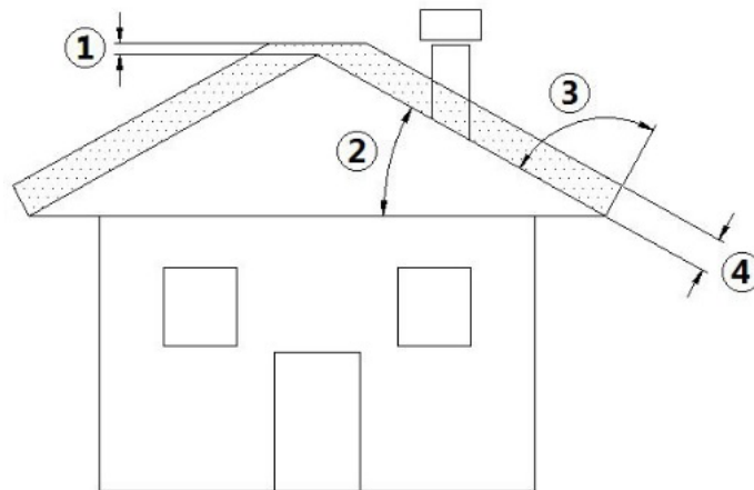
Fig. 3 - Geneigtes Dach
