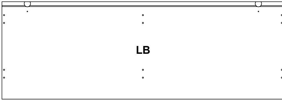
1157x399x18mm
