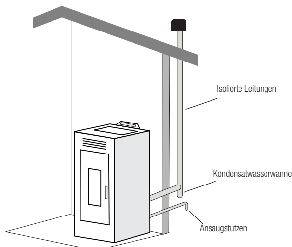
Bild 4: Installation des äußeren Schornsteins
