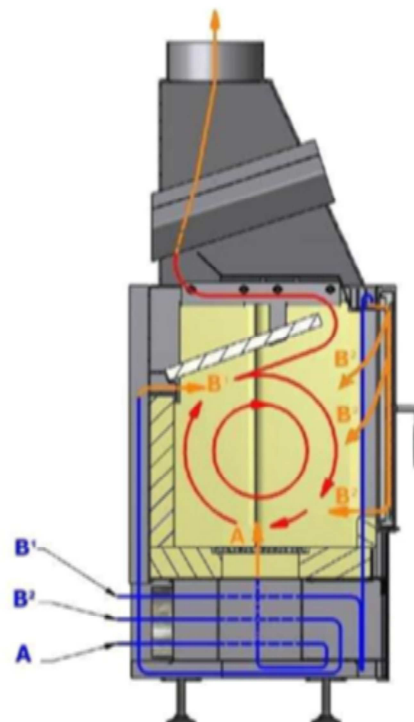
Abb. 1.7. Luftumwälzung
