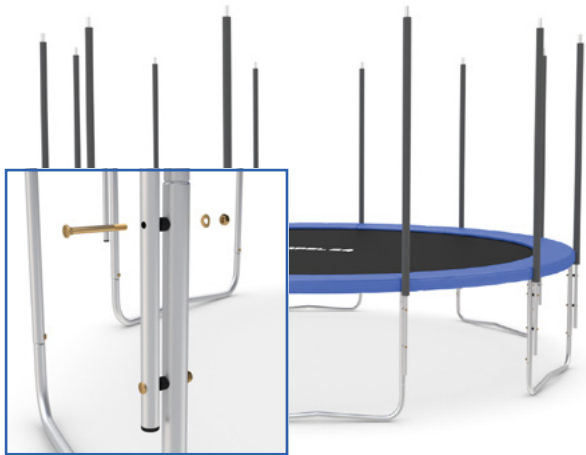
Abb. 4: Befestigung der Netzpfeosten
