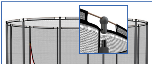
fig. 2: Assemblage du filet de sécurité aux montants
