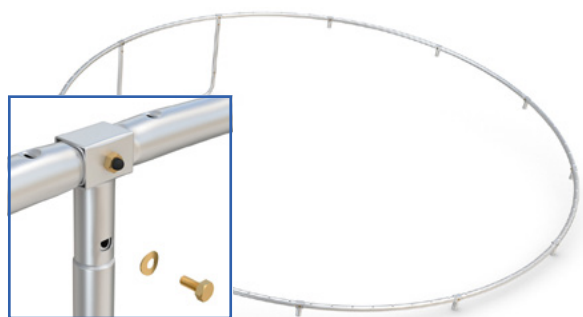
Abb. 4: Standfüße an den Rahmen schrauben
