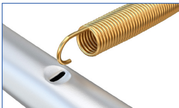
fig. 2: Fixation des ressorts au cadre tubulaire
