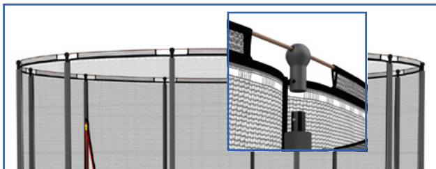
Abb. 2: Sicherheitsnetz mit den Netzpfeilern verbinden
