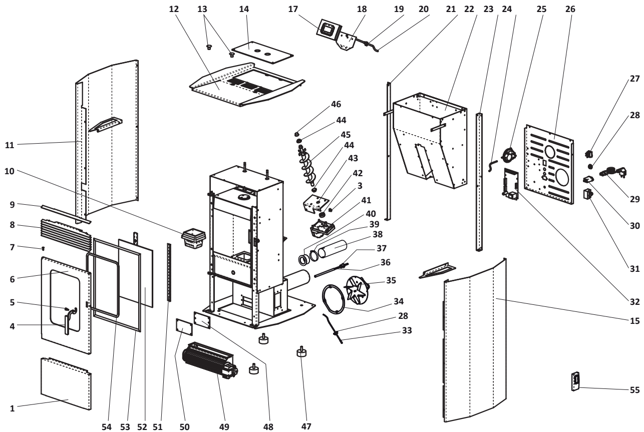
Abb. 14 Explosionszeichnung
