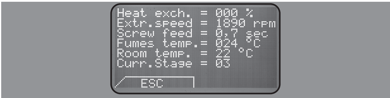
Abb. 10: Display-Anzeige im Info-Menü
