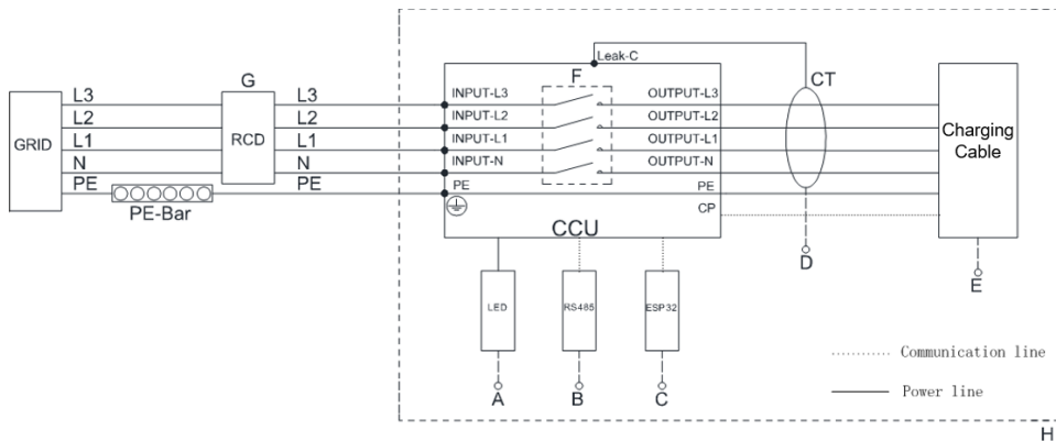
Abbildung 2-1 Schaltplan
