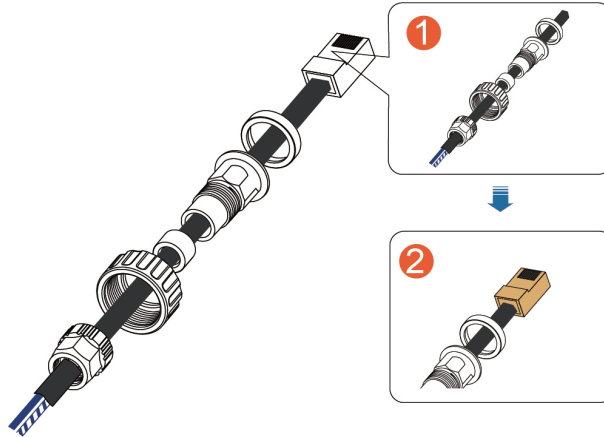
Abbildung 2-2 RJ45-Schraubanschluss (A)
