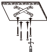
Per soffitti in legno
