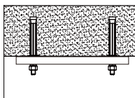
Per soffitti pieni
