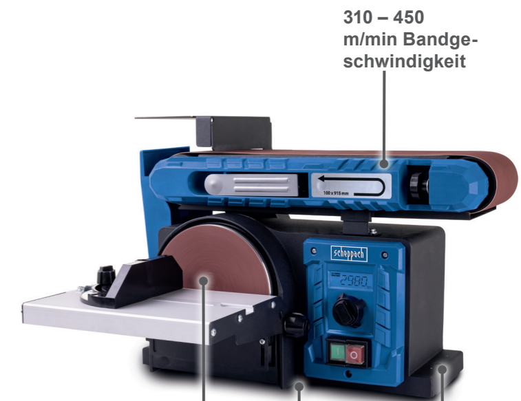
2000 – 2980 min -1 Schleifteller-geschwindigkeit
