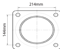
Baseplate SOLARIS PREMIUM
