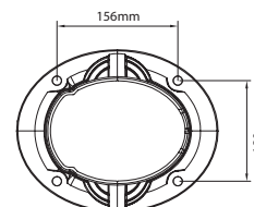
Bodenplatte SOLARIS LUXE
