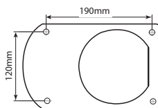
Baseplate SOLARIS XTRA
