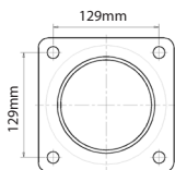
Vloerplaat SOLARIS PLUS
