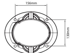
Baseplate SOLARIS LUXE
