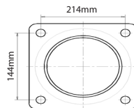
Plata de ducha SOLARIS PREMIUM
